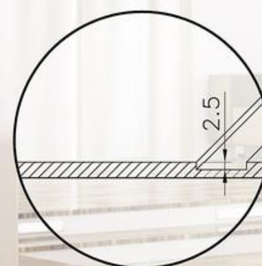
剖面厚度圖
