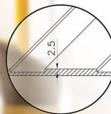
剖面厚度圖
